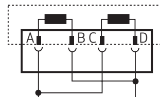
并联线圈
