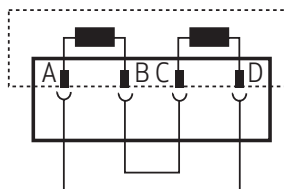
串联线圈
