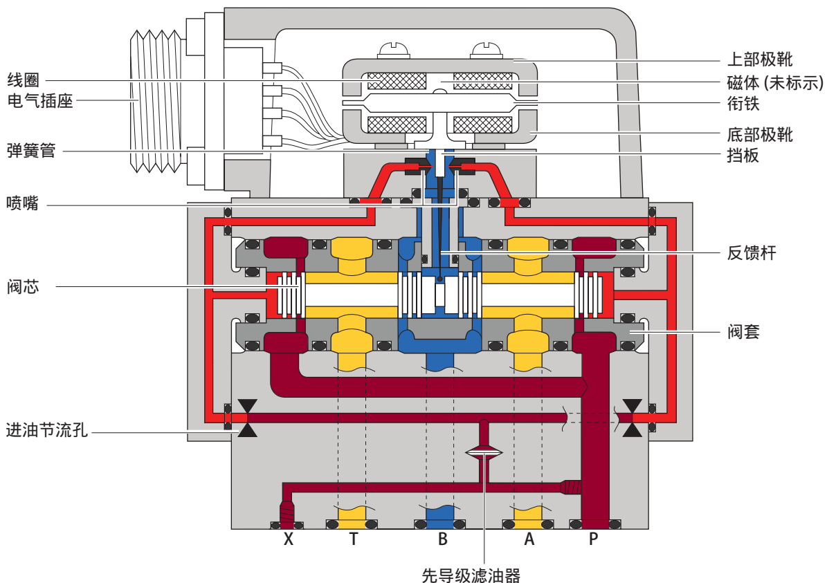
电液伺服阀剖视图
