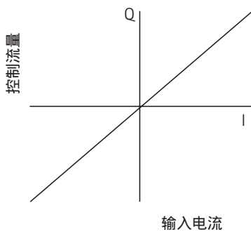
标准零遮盖
