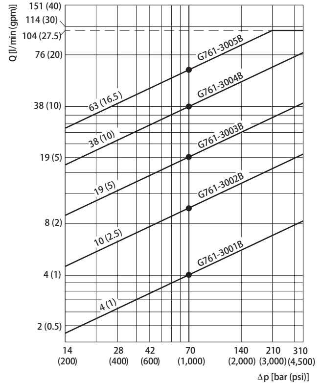
四通控制时的流量图
