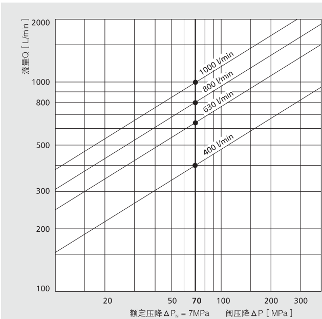
阀口全开 ( 100%给定输入信号 ) 时的伺服阀负载流量与阀压降的关系曲线
